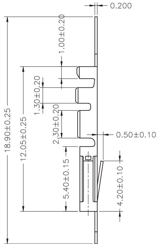
SEC:A-A
